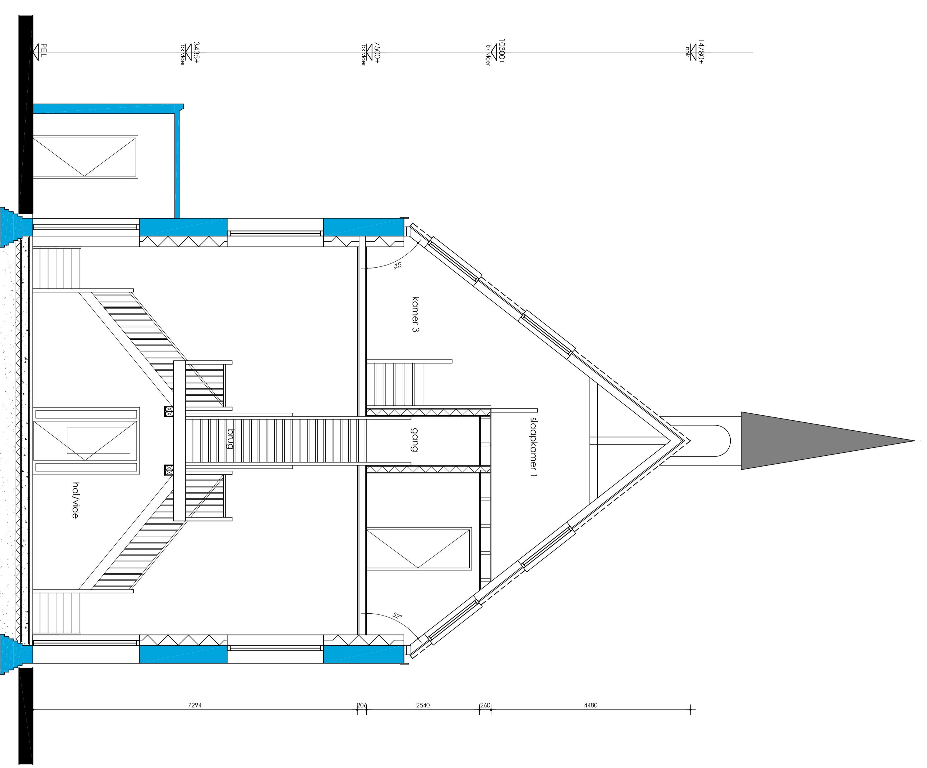
Doorsnede A-A
